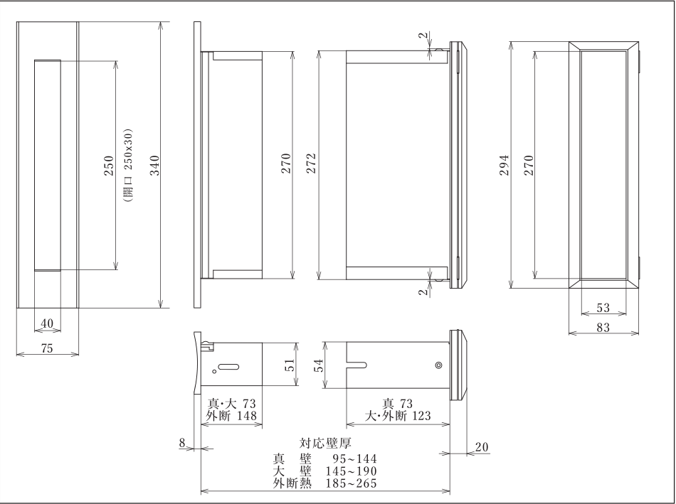
組み立て例
